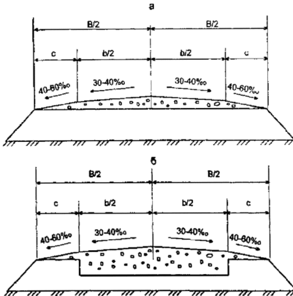
Рис. 1. Серповидный (а) и полукорытный (б) поперечные профили покрытий:
