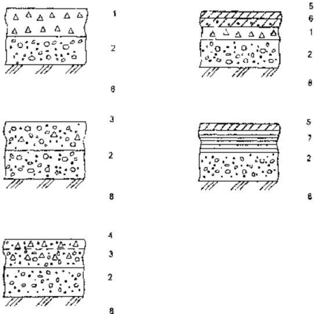
Рис 2. Конструкции дорожных одежд с покрытиями из щебеночно-гравийных материалов и отходов промышленности: 1 - щебень; 2 - готовая гравийно-песчаная смесь оптимального зернового состава или песок; 3 - готовая щебеночно-гравийно-песчаная смесь; 4 - то же, обработанная обеспыливающими материалами; 5 - поверхностная обработка или слой износа из мелкозернистого асфальтобетона; 6 - щебень, обработанный неорганическими вяжущими; 7 - отходы промышленности; 8 - грунт земляного полотна
